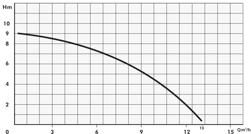
Obr.1. Závislosť prietoku v m³ za hodinu od výtlačnej výšky v metroch.
