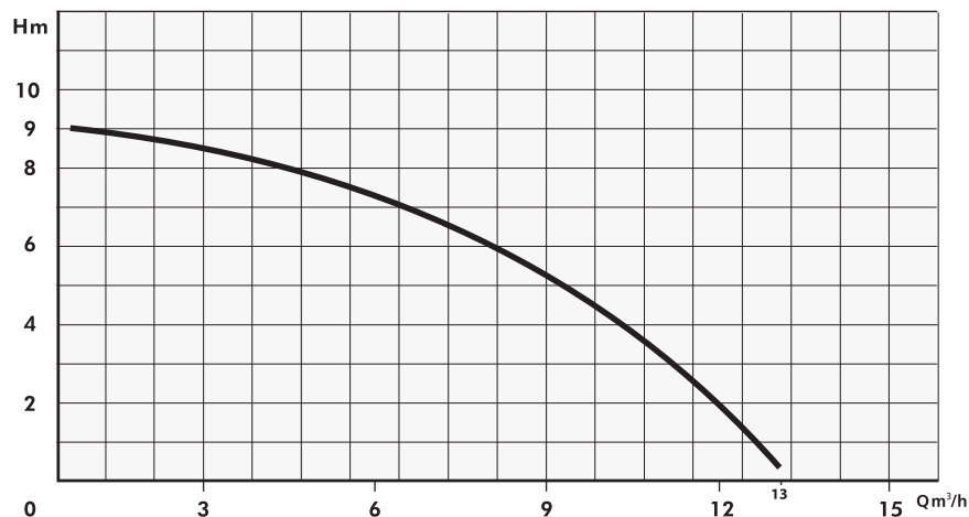
Abb. 1, Abhängigkeit des Durchflusses in m³ pro Stunde von der Druckhöhe in Metern.
