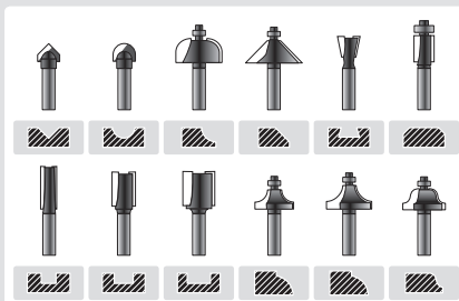
Abb. 1, Profilform in Abhängigkeit vom eingesetzten Formfräser
