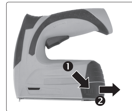
4. ábra. A kapocs/szeg adagoló kihúzása
