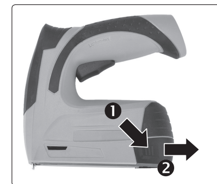
Obr. 4, vysunutí posuvníku spon/hřebíků
